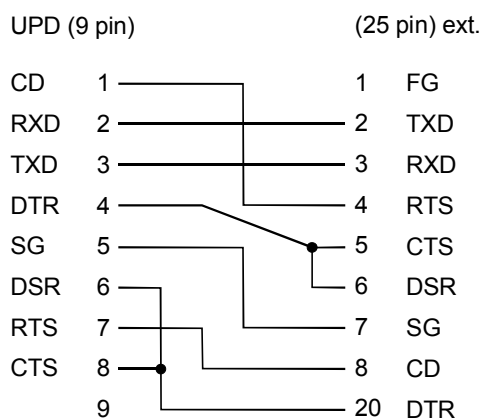
Bild 2-45 25-polige serielle Schnittstelle
