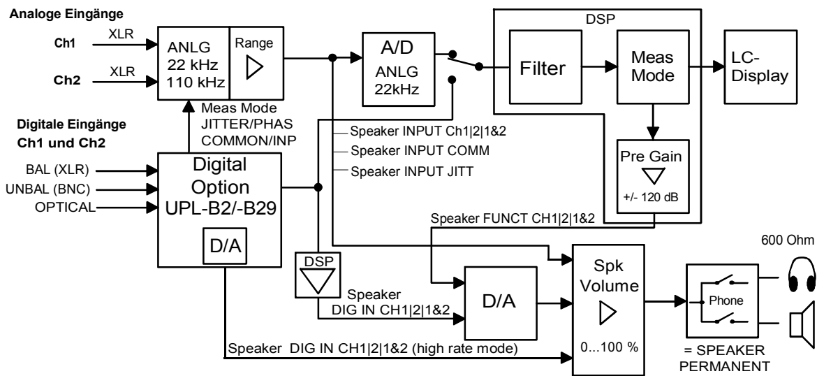
Bild 2-28 Funktionsprinzip des Mithöerausgangs
