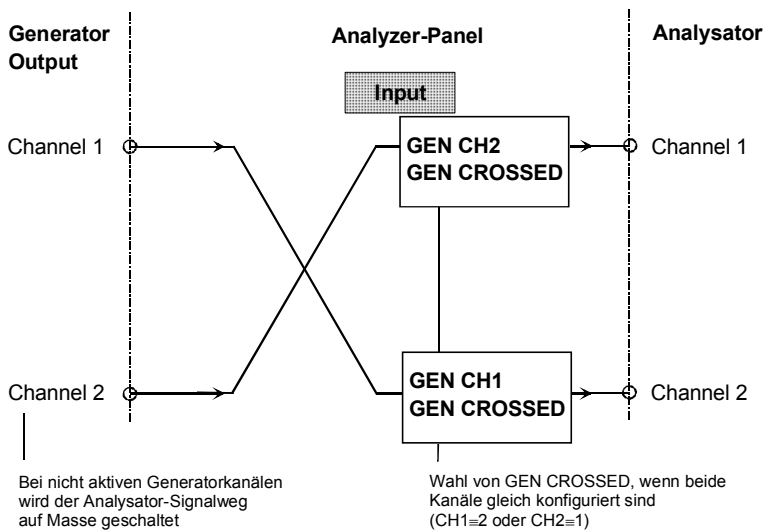
Bild 2-19 Interne Signalwege
