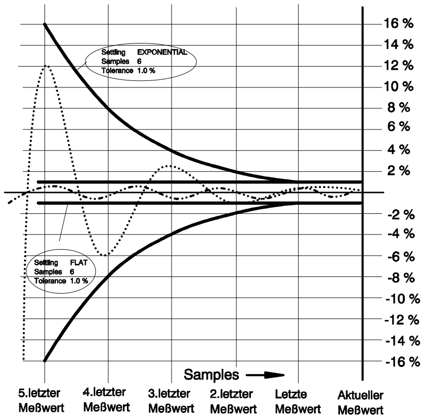
Bild 2-9 Toleranzverlauf
