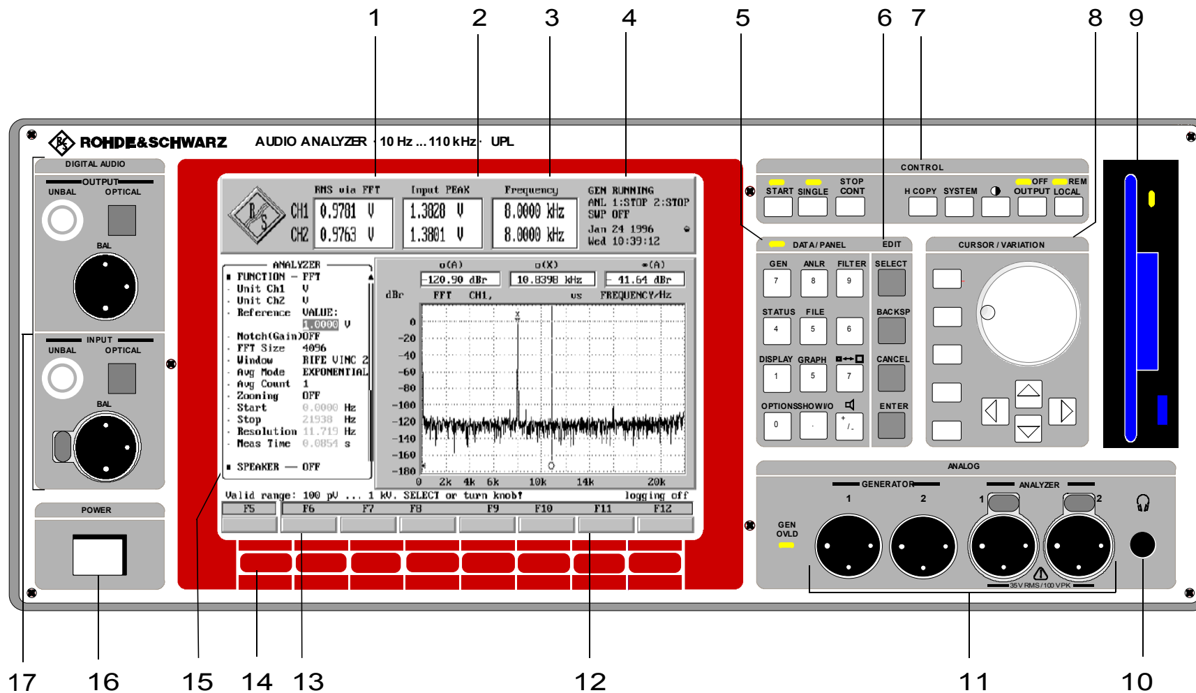
Bild 2-1 Frontansicht
