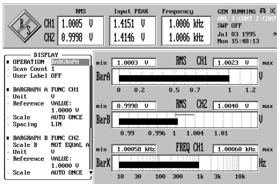
Bild 2-41 Bargraph-Darstellung
